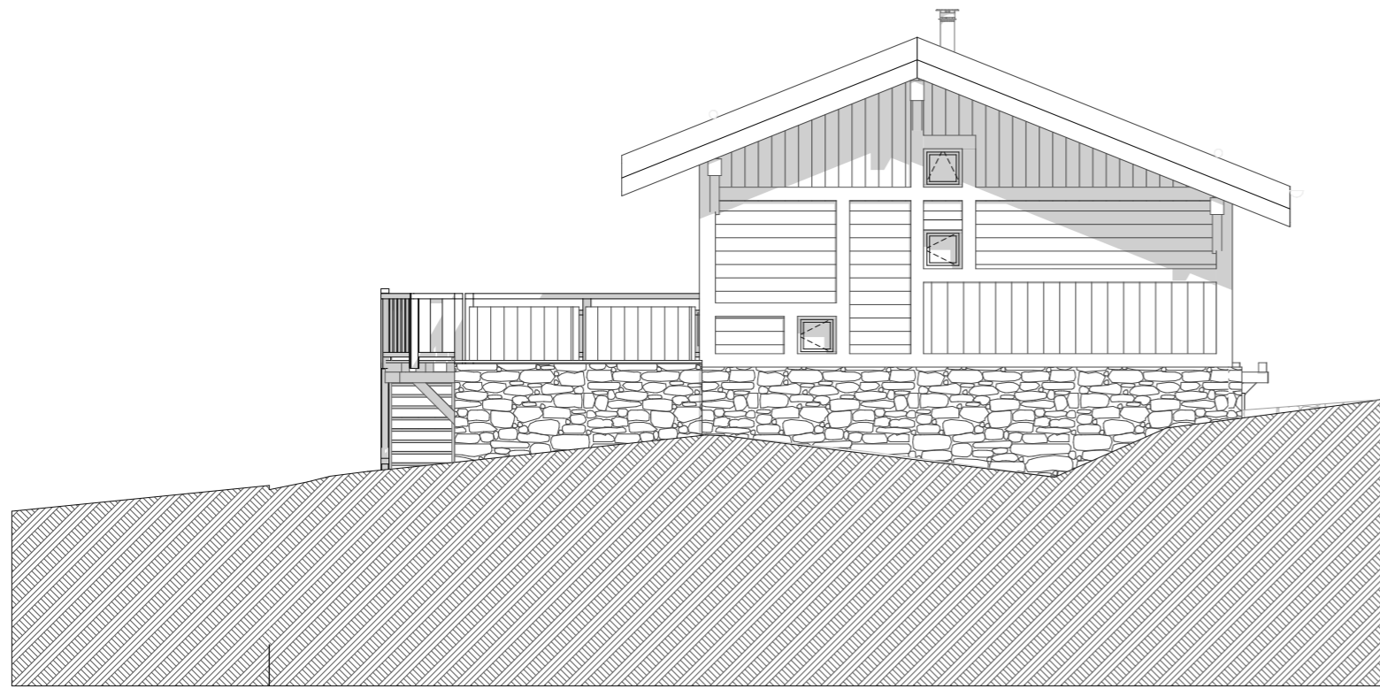
Façade Nord-Ouest
