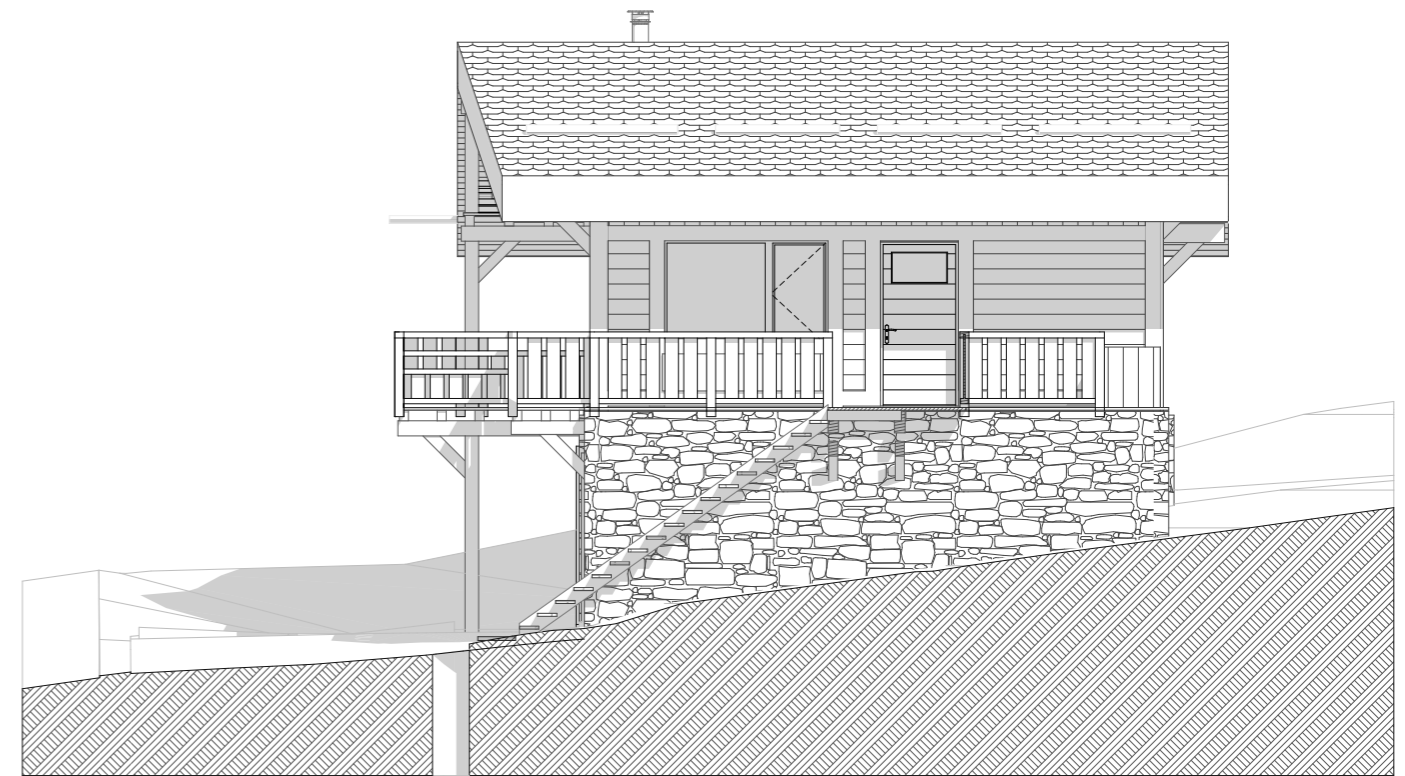
Façade Nord-Est
