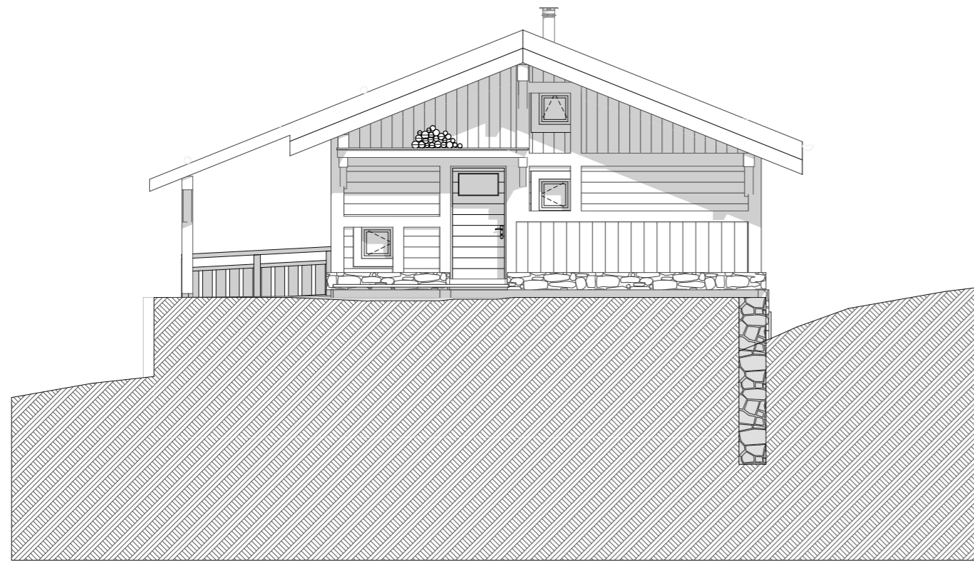
Façade Nord-Ouest
