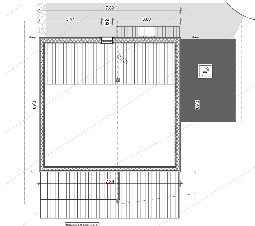
1:100 Deuxième étage 2.
