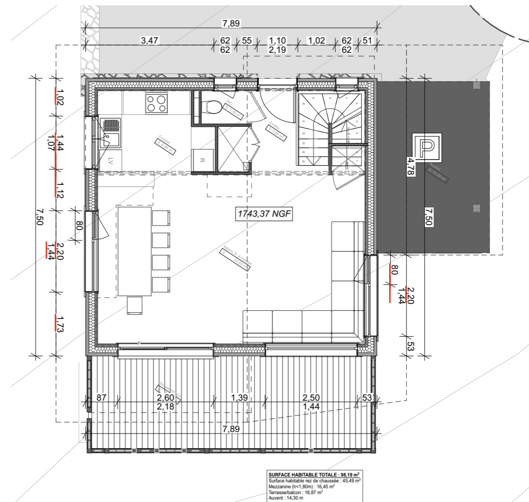
1:100 Premier étage 1.
